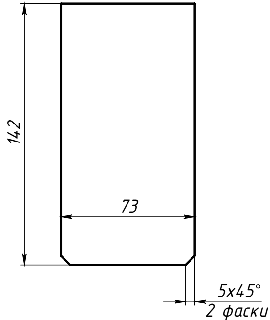
Поз.2 (Ребро)
